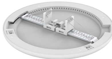
Ajustable au trou/Adjustable to hole: Ø 65-205mm
